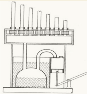
Coupe de l'orgue hydraulique de Ctésibios décrit par Héron d'Alexandrie (mathématicien grec, 1er siècle après J.C.). Une seule pompe, une seule rangée de tuyaux.
